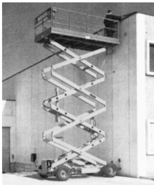
Figura 6 Esempio di piattaforma mobile
